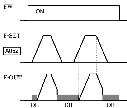
Ex.2) Cambio analógico en F-SET.
