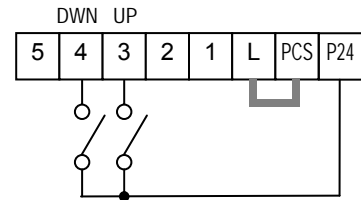
Especificación de terminales en pág. 4-6 .
