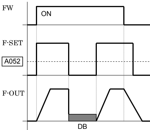
Ex.1) Cambio en F-SET.
