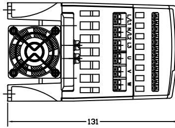
VISTA INFERIOR
